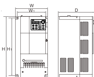
图 C-6 框架 D 安装尺寸
