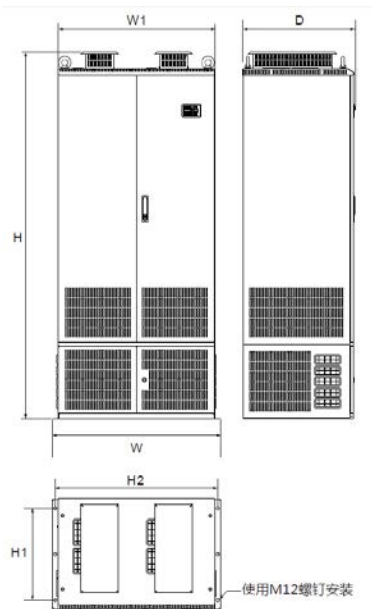
图 C-11 框架M安装尺寸
