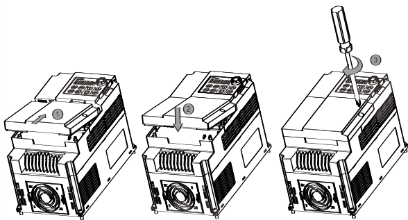
图 2-8 端子盖的安装
